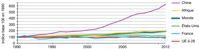
Émissions de CO 2 dues à la production d'électricité dans le monde 1
