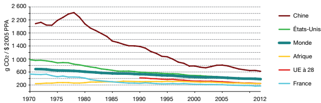
Émissions de CO 2 dues à l'énergie par rapport au PIB dans le monde
